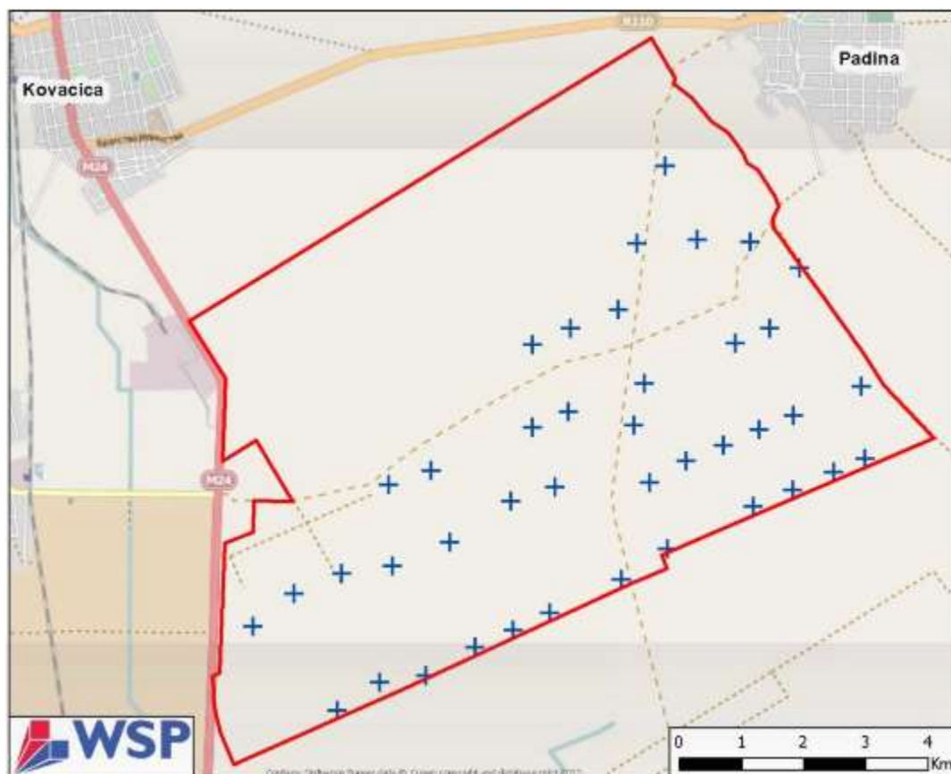
Slika 2 – Situacioni plan vetrogeneratora u okviru otiska Projekta
